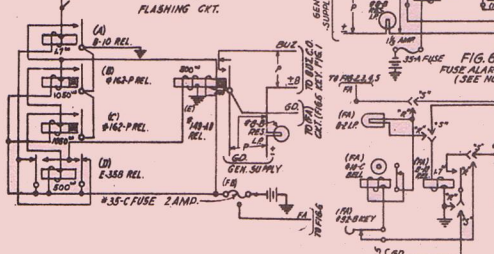
FIG. 5 FLASHING CKT.
