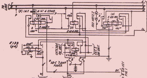
FIG. 3 INTERCEPTING LINE CKT.
