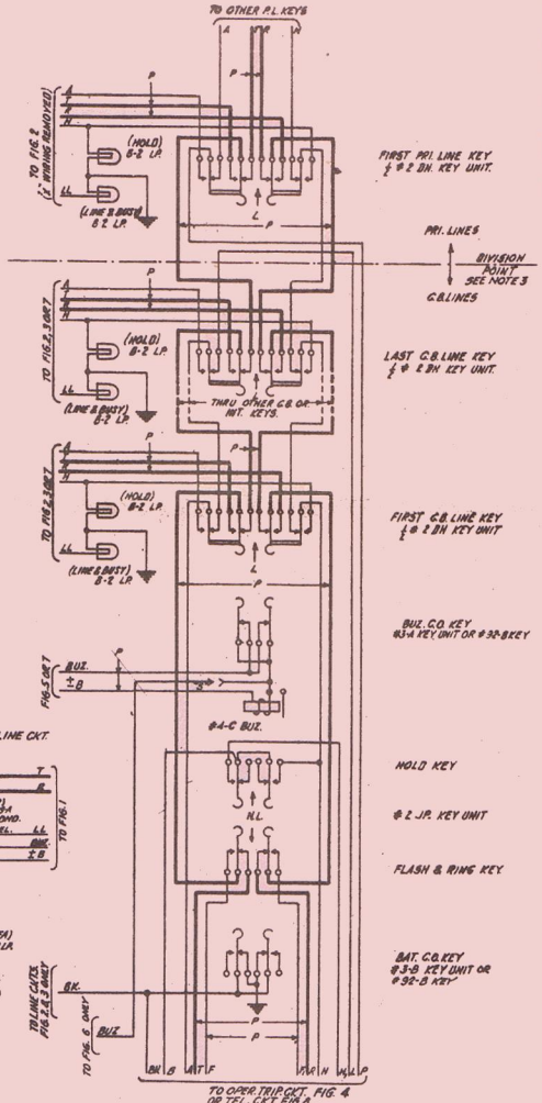
FIG. 1 TURRET WIRING
